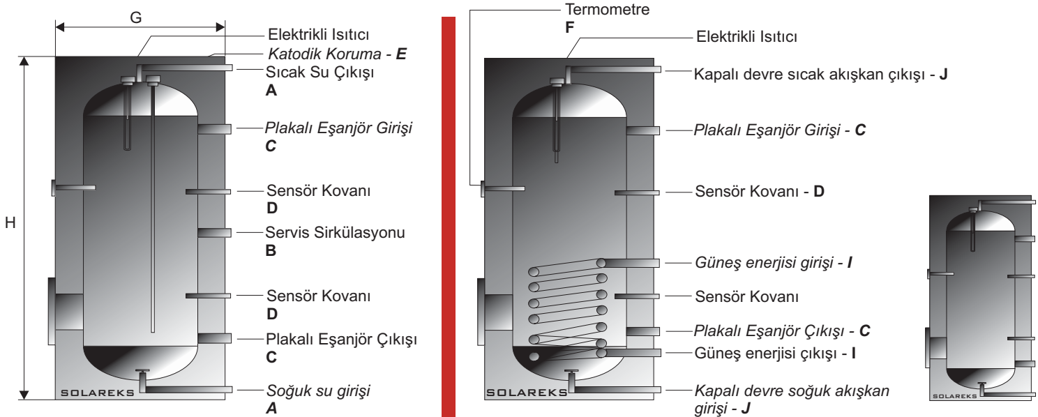
Kullanım suyu akümülyasyon tankı
